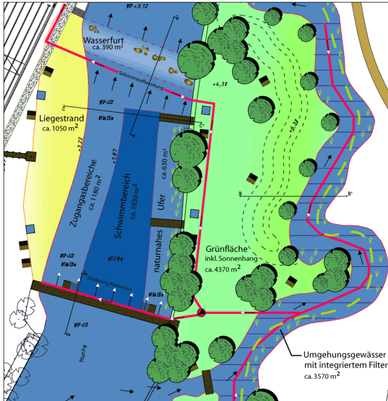
Entwurfsplanung Flussbad Mühlhunte, Oldenburg Quelle: Polyplan GmbH, Bremen 2004
